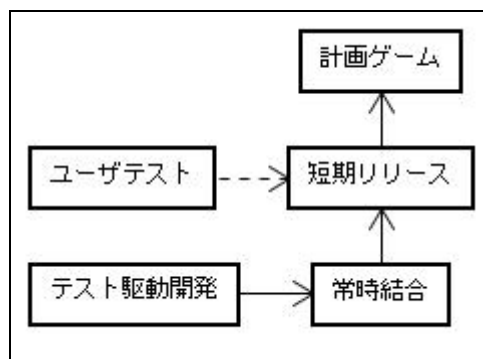
図4 要求品質向上のプラクティス群
