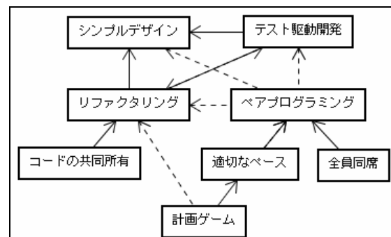
図 2 生産性向上のプラクティス群
